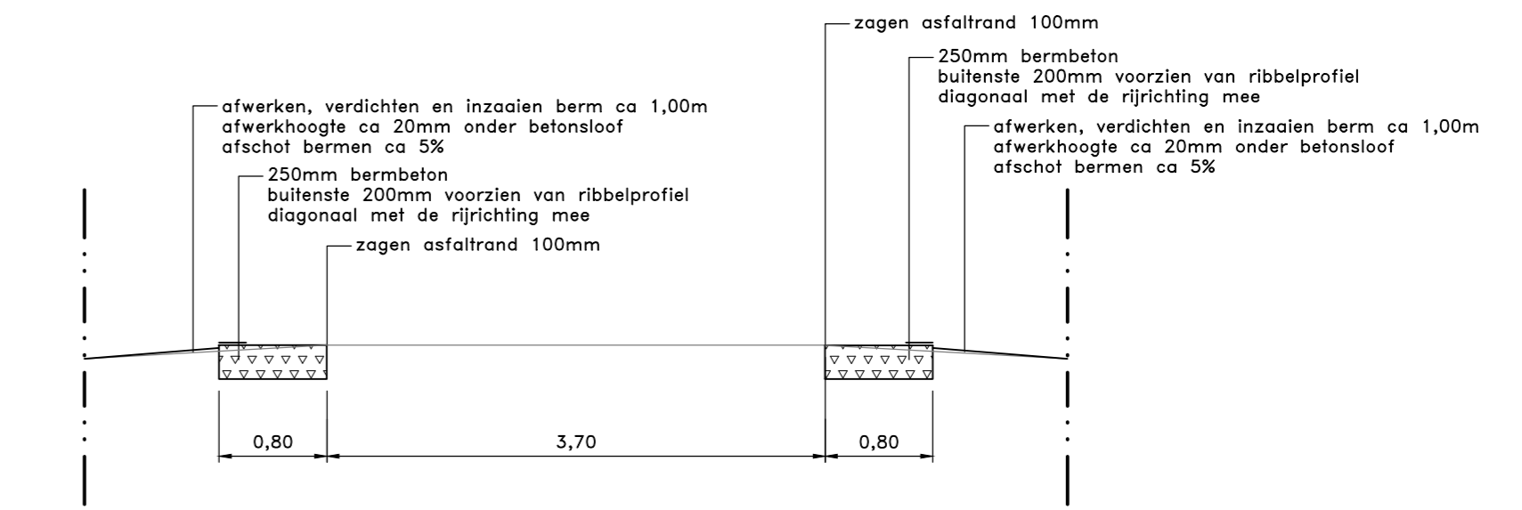
Principeprofiel E-E
