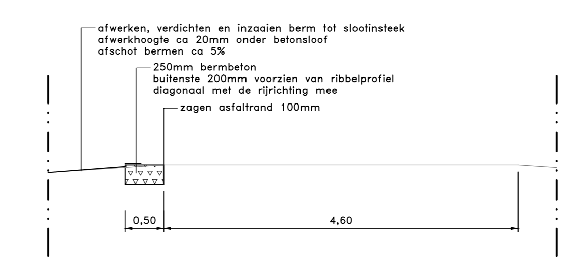
Principeprofiel D-D
