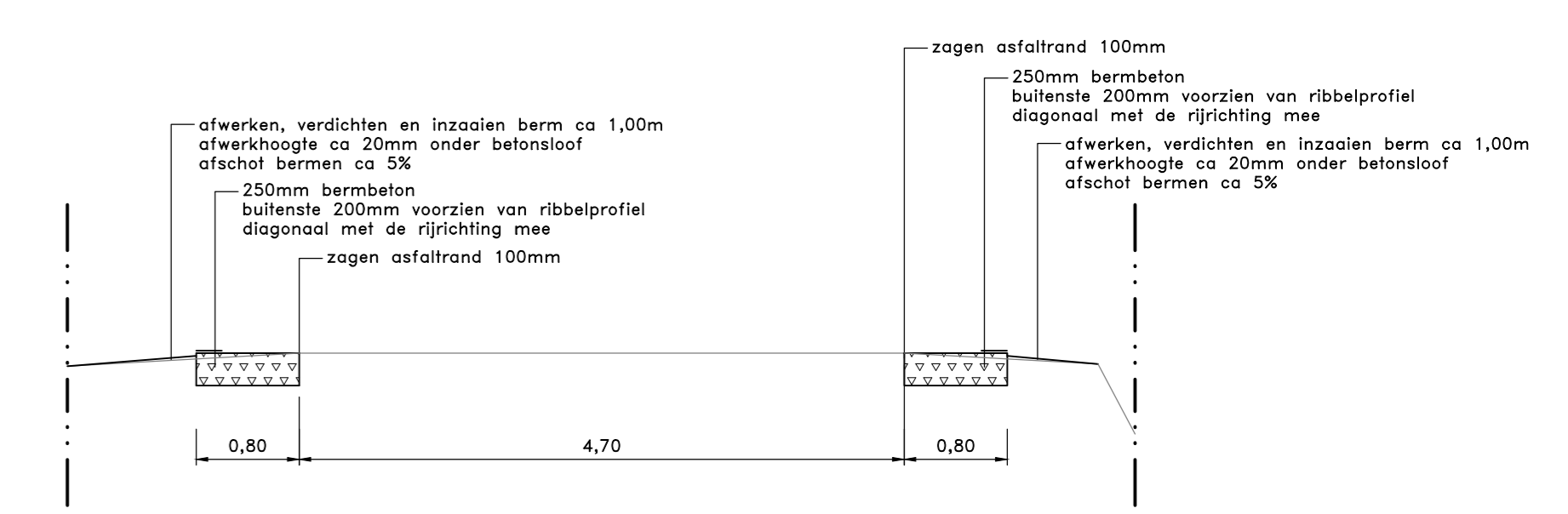
Principeprofiel H-H schaal 1:50
